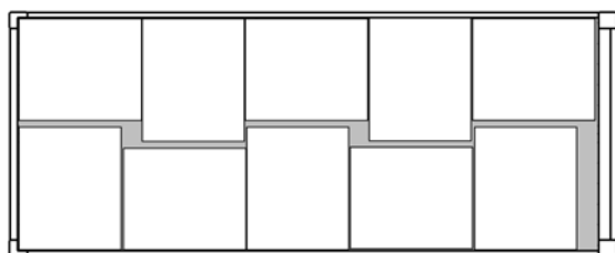
Figure 7.29 - Chargement d'unités de charge de 1 000 x 1 200 mm dans un conteneur de 20 pieds (6 mètres)
