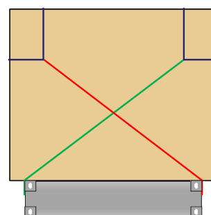
Figure 7.48 - Saisine à ressort transversale
