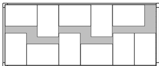
Figure 7.30 - Chargement d'unités de charge de 800 x 1 200 mm dans un conteneur de 20 pieds (6 mètres)
