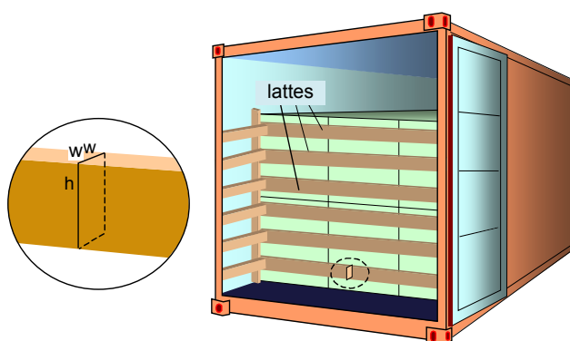
Figure 7.6 - Disposition générale des barres de clôture dans un engin de transport pour protéger la porte
