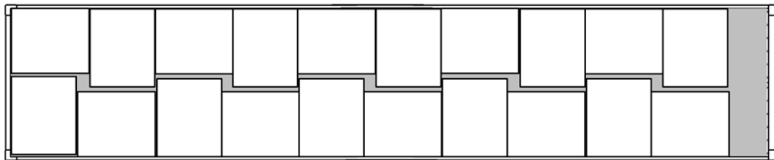
Figure 7.31 - Chargement d'unités de charge de 1 000 x 1 200 mm dans un conteneur de 40 pieds (12 mètres)
