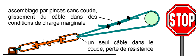
Figure 7.15 - Mauvais assemblage de saisine en câble métallique
