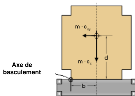
Figure 7.37 - Critère de basculement
